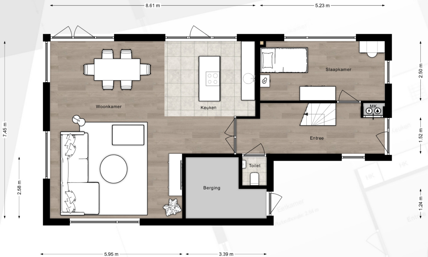
Bouwnummer 7 Begane grond
